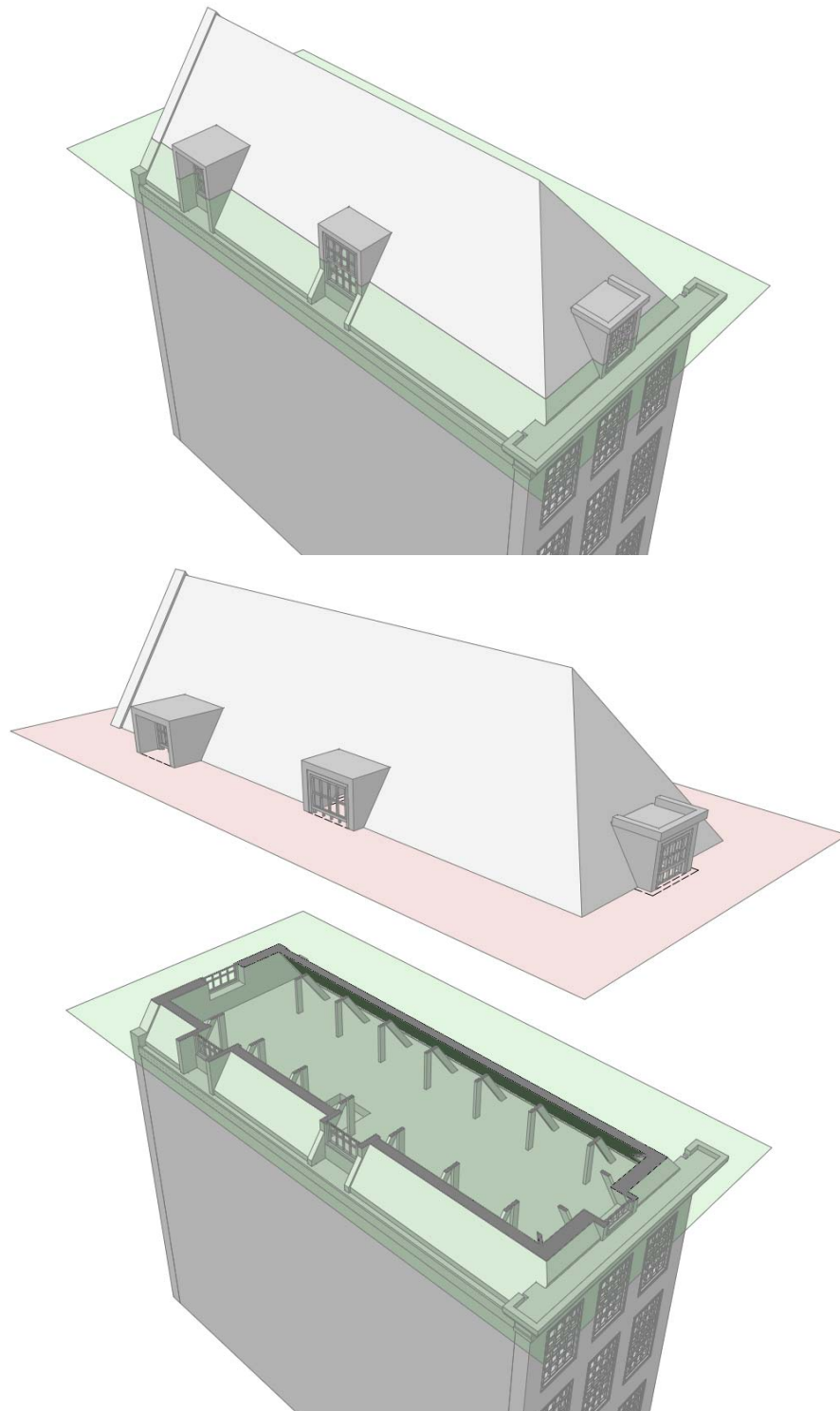
Figuur 2: projectievlak aangebracht: lichtgroen vlak voor componentdoorsnijing, roze voor componentprojectie.
